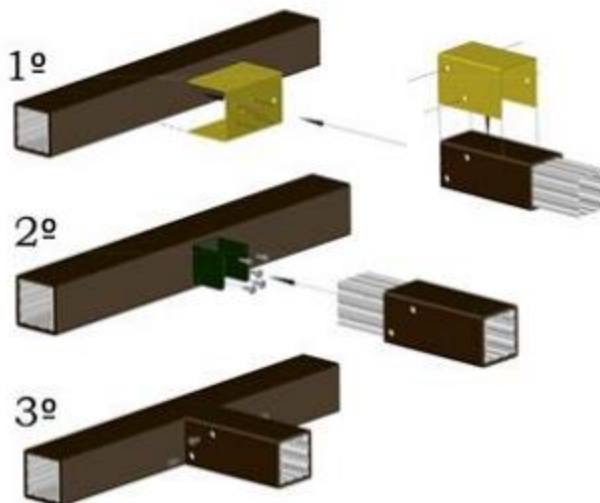
Conexión 90°
